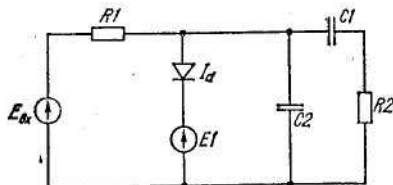
Рис. 8.7. RC-схема
