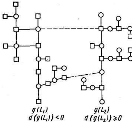
Рис. 10.9. Членение остова информационного графа на критическое множество и множество без дефицита (— — — — ребра, удовлетворяющие условию (10.44); — . — . — — ребра, не удовлетворяющие условию (10.44); □ — вершины-переменные; ○ — вершины-связи)
