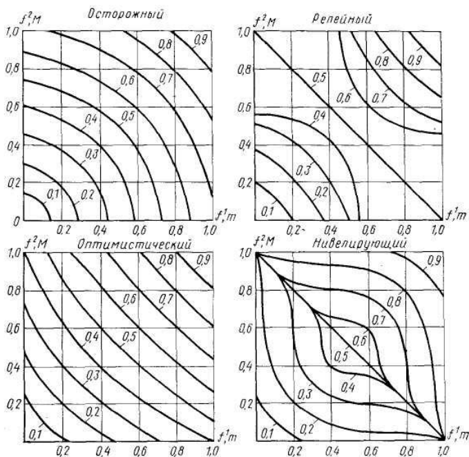
Рис. 10.57. Номограмма для вычисления n -обобщенных потерь при отдельных способах учета неопределенности по Mm — методу или при оценке рекомендации двумя критериями f^1, f^2 .
