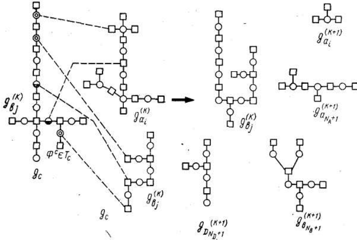
Рис. 10.18. Выполнение оператора КС (●- элементы \Phi^6 ;
