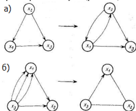
Рис. 8.17. Преобразование графов
