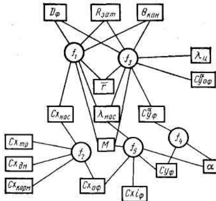
Рис. 10.5. Пример неориентированного двудольного информационного графа модели (□ — вершины-переменные, ○ — вершины-связи)
