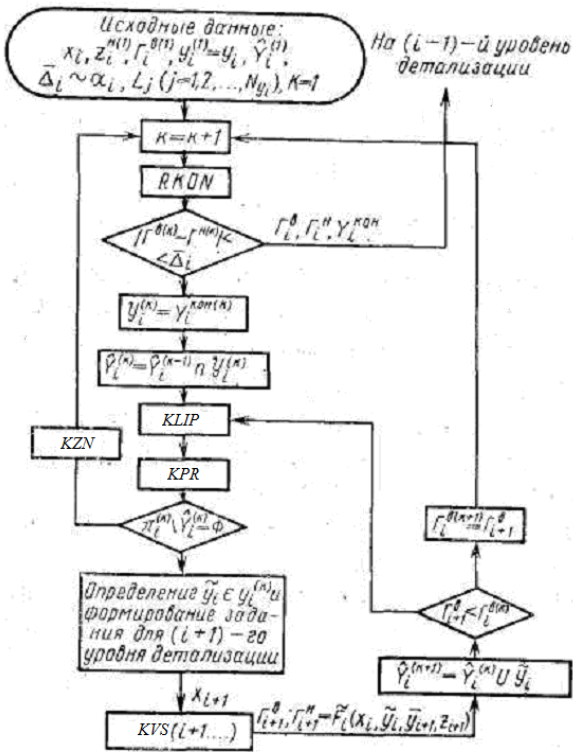
Рис. 10.32. Структура алгоритма формирования конкурентоспособных рекомендаций на i -м уровне детализации формируемых рекомендаций
