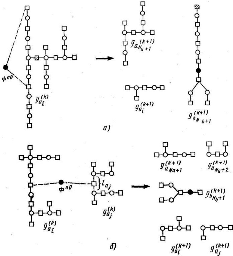
Рис. 10.12. Выполнение оператора KOO(a) \sigma^{a0} \subseteq g_{a_i}; \sigma^{a0} \subseteq g_{a_j}
