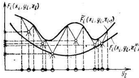
Рис. 10.30. Определение липшицевых точек (● — соответствует \hat{Y}_i ; ● — соответствует Y_{li} ; ○ — соответствует l_i )
