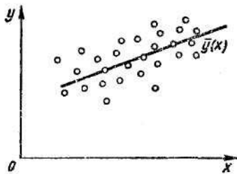
Рис. 9.8. Линия регрессии
