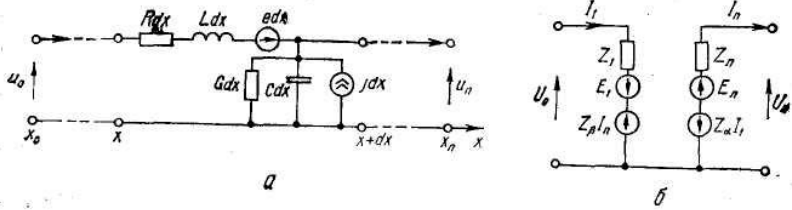
Рис. 8.4. Схема замещения длинной линии: a — многосекционная, б — эквивалентным четырехполюсником
